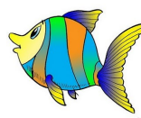
PEIXE
