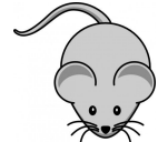
RATO
